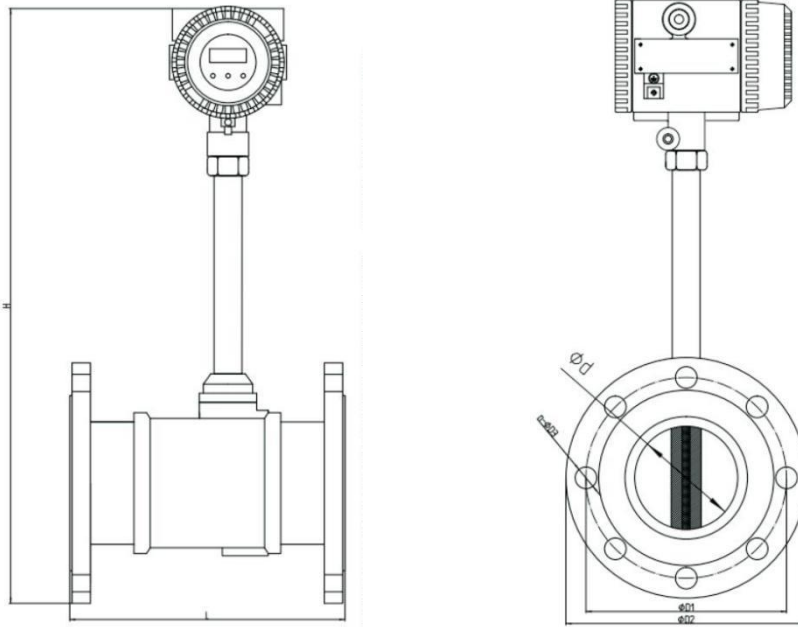
DIN PN16 Flange Connection Dimension
